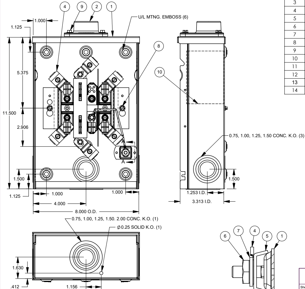
SECTION A-A SCALE 1 : 1
